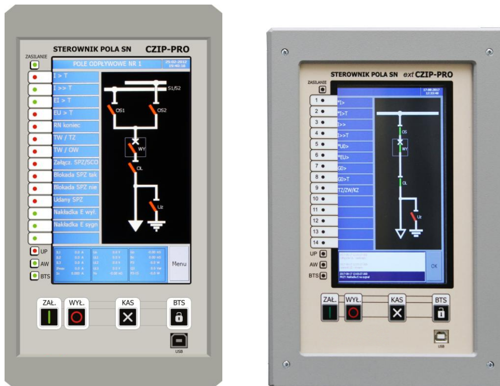
Rys. 9.1. Widok płyty czołowej zespołu CZIP-PRO i extCZIP-PRO
